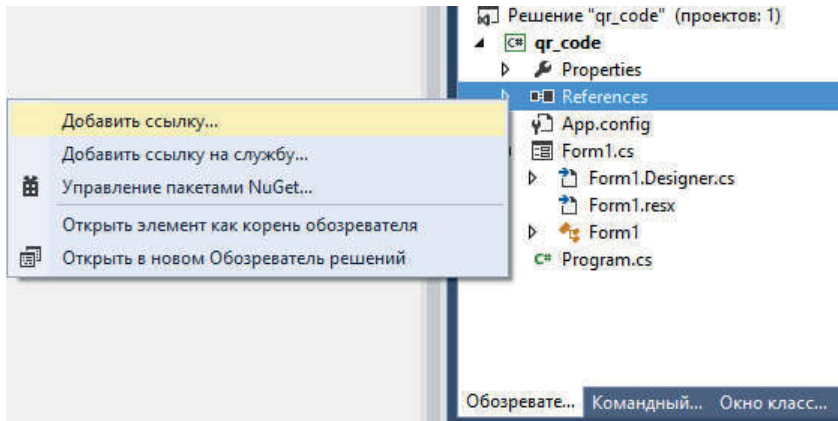
Рис. 3. Подключение библиотеки для работы с QR-кодами на C#
